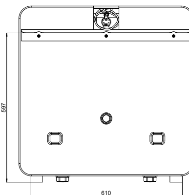
Vista posteriore
