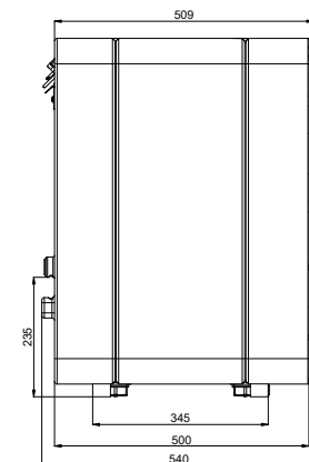
Vista laterale
