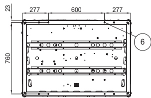
DISPOSIZIONE FORI MONTAGGIO (VISTA DAL BASSO) MOUNTING HOLES LOCATION (BOTTOM VIEW)
