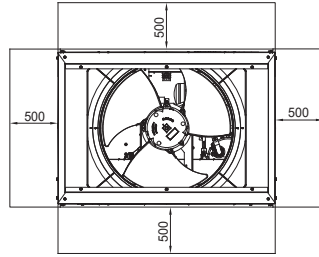
SPAZIO MINIMO NECESSARIO MANUTENZIONE MINIMUM REQUIRED MAINTENANCE
