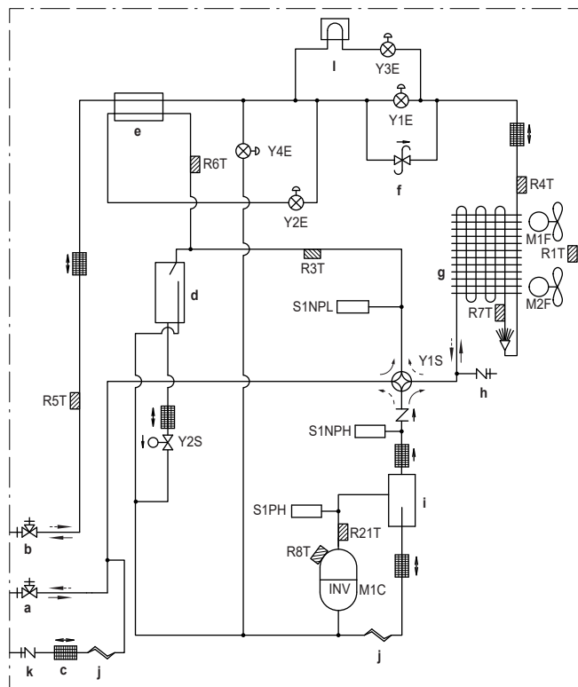
Schema delle tubazioni: 10+12 HP
