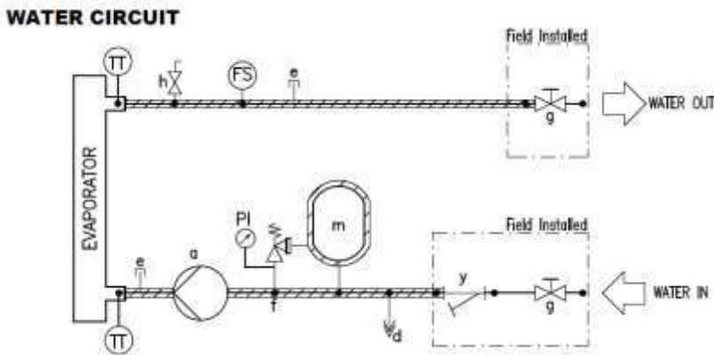
Figura 13 – Schema idraulico
