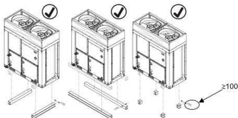
Figura 4 – Posizionamento dell'unità MONO
