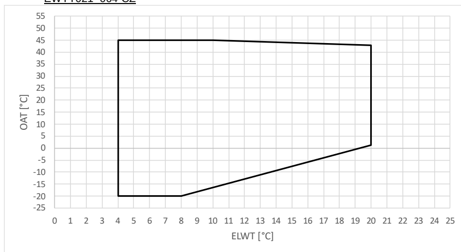
Figura 17 – Limiti operativi su EWYT_CZ nella modalità di raffreddamento
