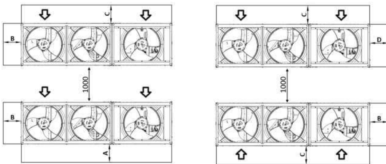
Figura 9 – Unità installate affiancate lungo i lati più lunghi (caso 1 e caso 2)
