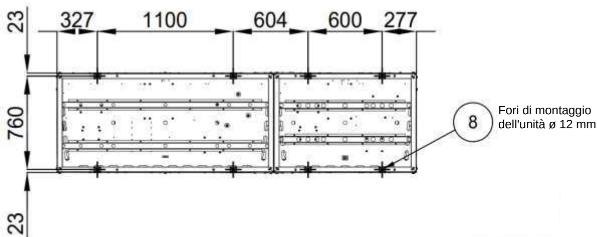
Figura 6 – Posizione dei fori di montaggio (vista dal basso)
