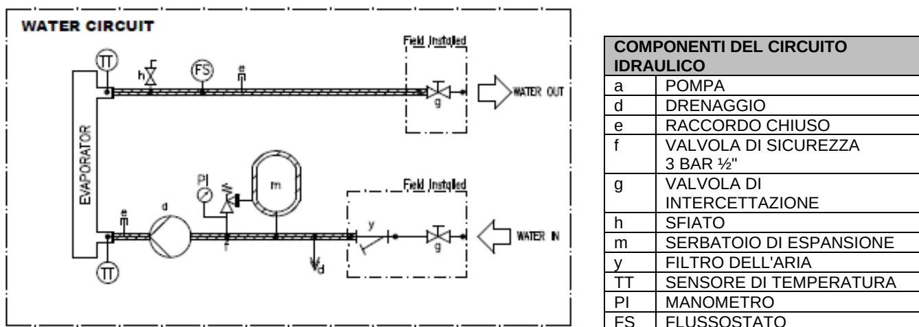
Figura 25 – Schema P&ID del circuito idraulico per unità EWYT-CZ
