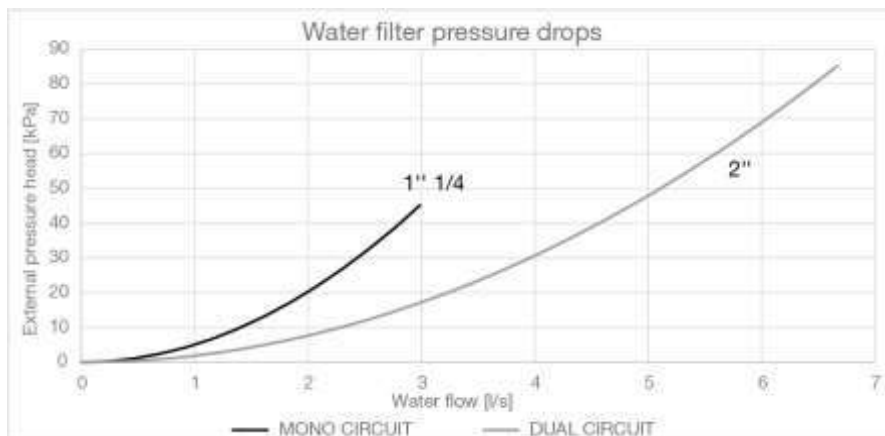
Figura 15 – Cadute di pressione del filtro dell'acqua
