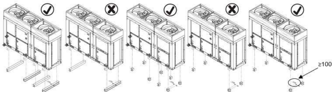
Figura 5 – Posizionamento dell'unità DUAL
