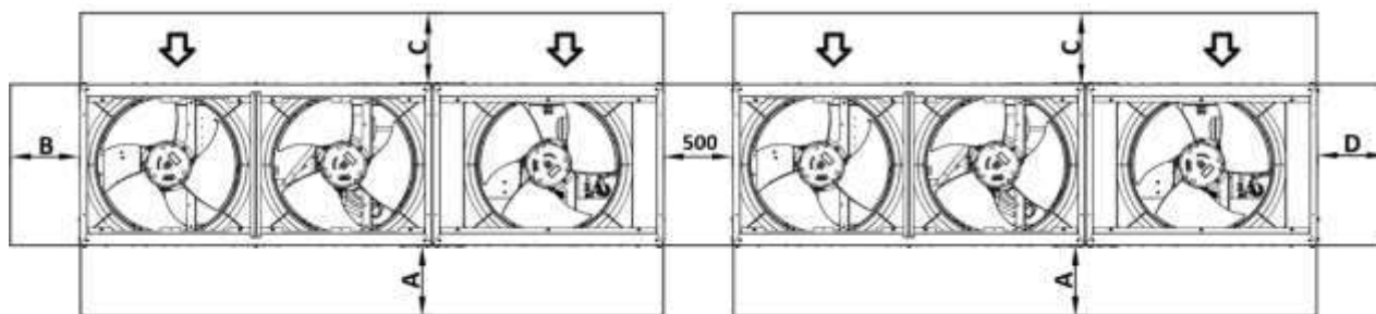
Figura 8 – Unità installate affiancate lungo i lati più corti, B o D
